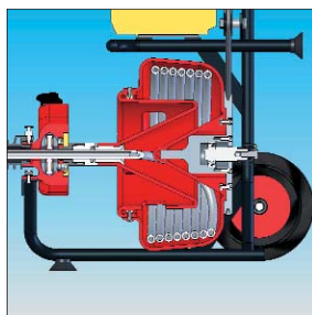
Защита спирали благодаря принудительному направлению в барабане
