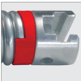
Фиксирующее кольцо из эластичного, самозакрывающегося материала
