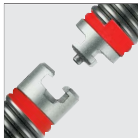
Самостопающееся соединения спирали и муфты
